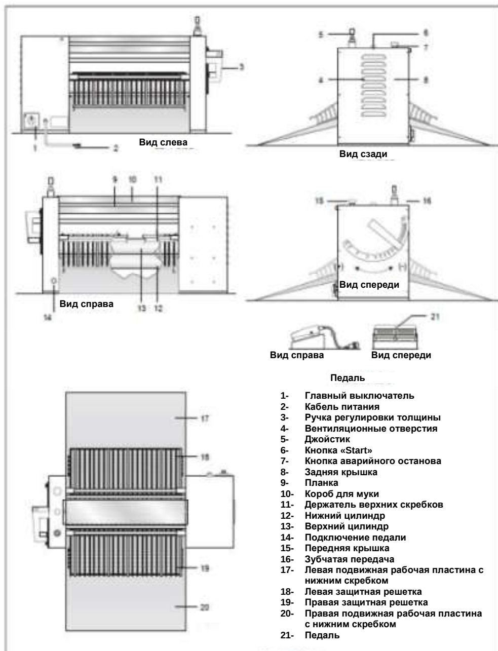
Рис.1 (компоненты машины)
