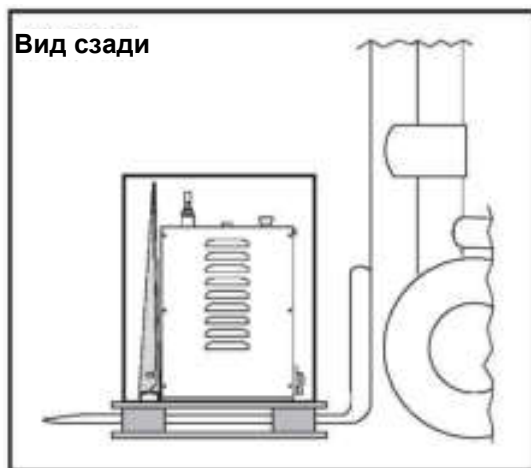
Рис.4 (Подъем упаковки вилочным погрузчиком)
