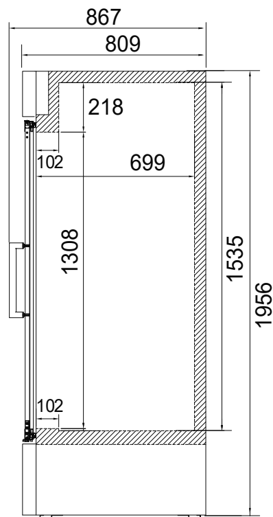
ВИД СБОКУ
