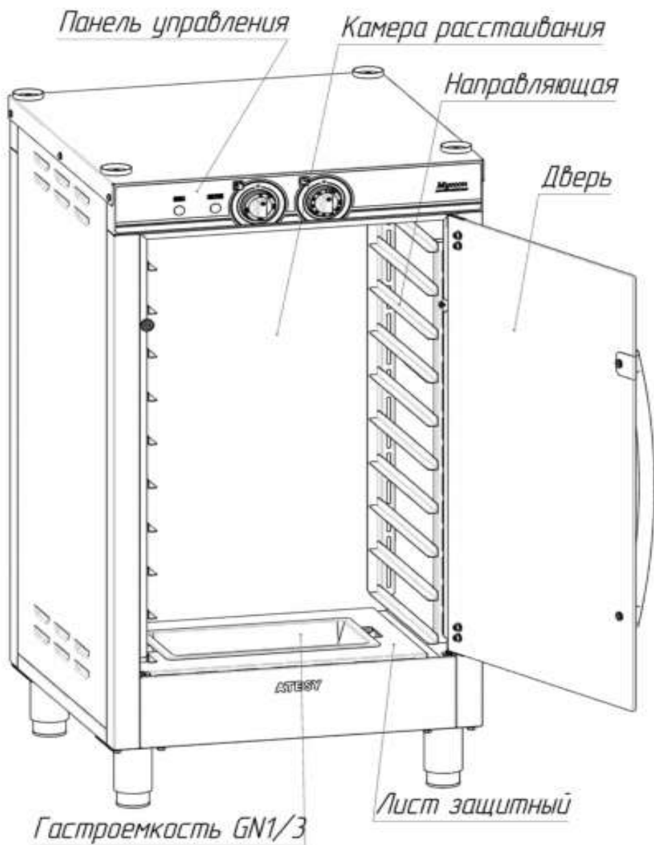
Рис. 1. ШР-10-430.330-01.
