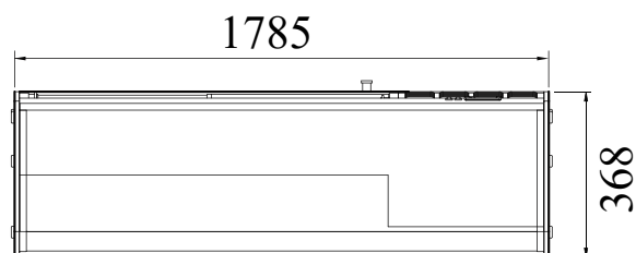
ВИД СВЕРХУ
