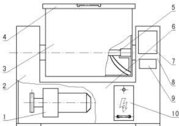
Рис. 1-1 Деталировка BWL-100
