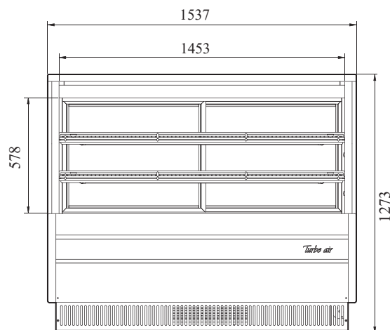
ВИД СПЕРЕДИ
