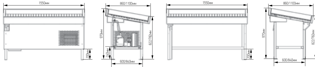
выносное холодноснабжение
