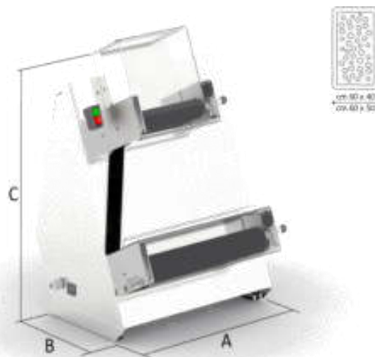
Рис. 2.7.2. - Тестораскаточная машина для пиццы SPR 30 PA / SPR 50 PA
