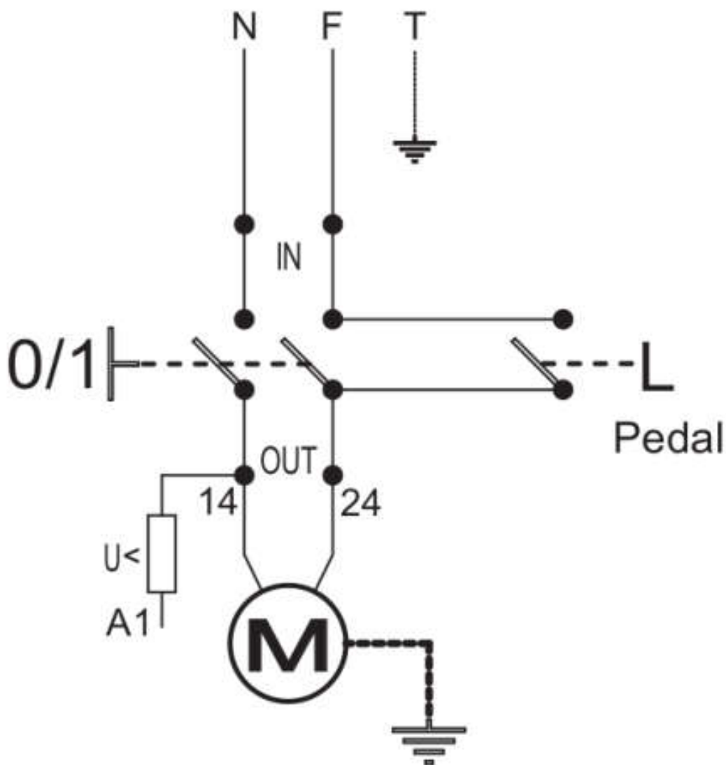
Рис. 8.1. – Электрическая схема
