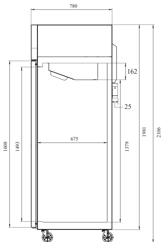
ВИД СБОКУ
