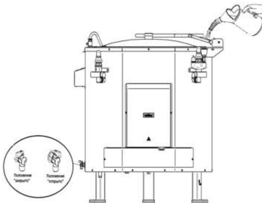
Рисунок 3 Залив воды в «рубашку»
