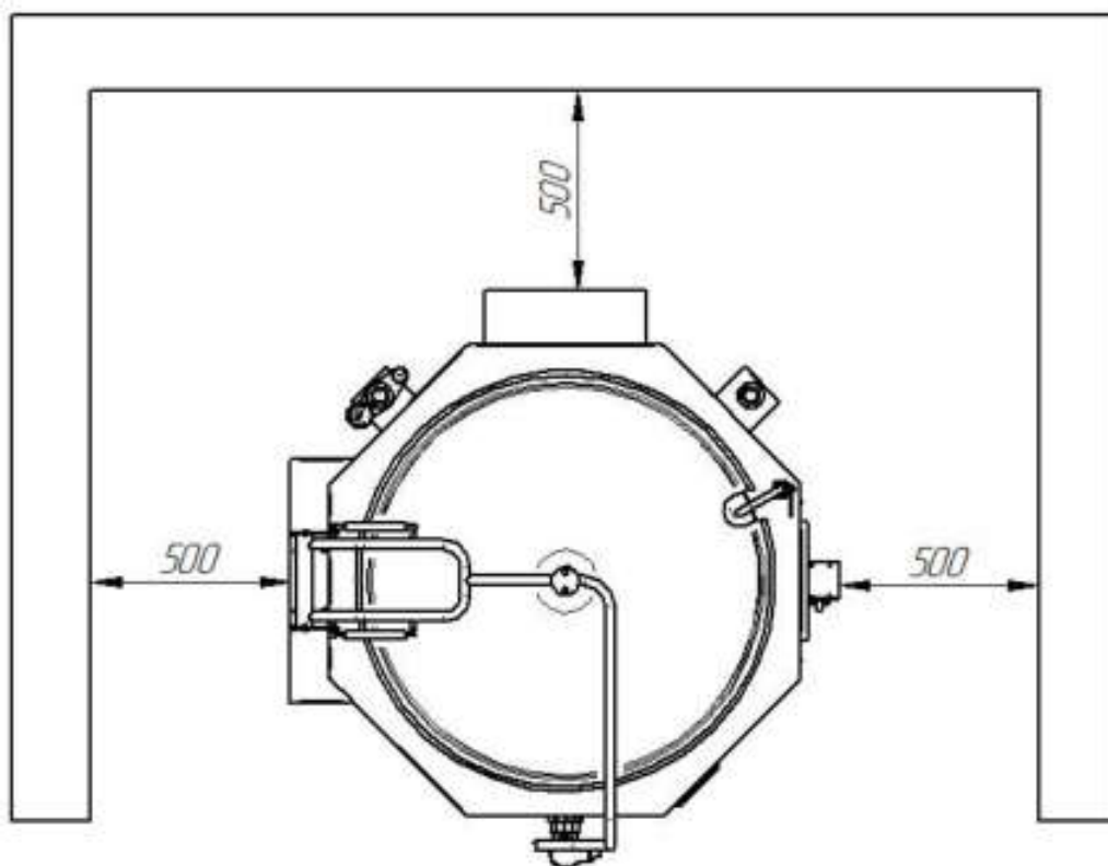
Рисунок 2 Установка котла
