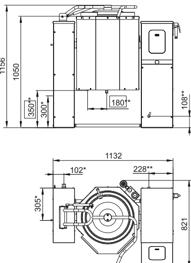
КПЭМ-60-0
