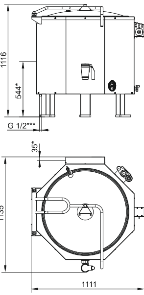
КПЭМ-250
