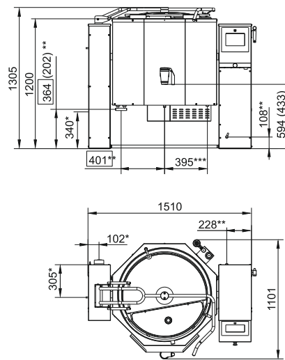
КПЭМ-250-ОМП, КПЭМ-350-ОМП (с краном)
