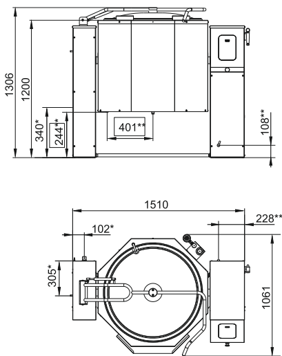
КПЭМ-350-О
