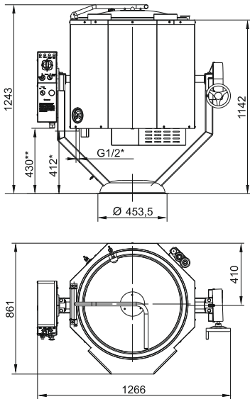
КПЭМ-160-ОМР
