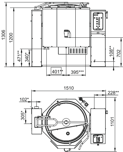
КПЭМ-200-0М2 (с краном)
