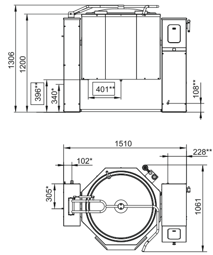
КПЭМ-250-0
