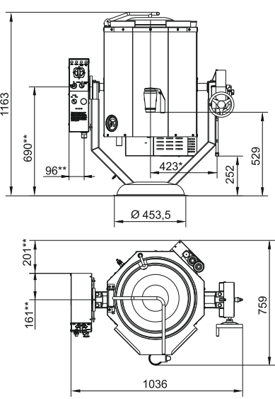
КПЭМ-60-ОМР
