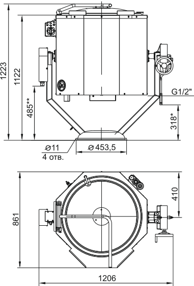
КПЭМ-160-ОР
