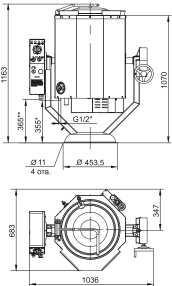
КПЭМ-60-ОМР
