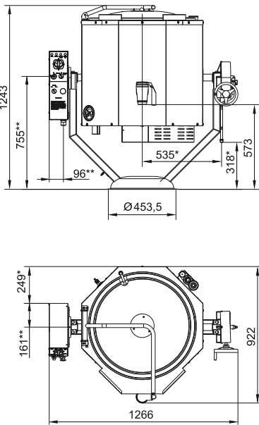
КПЭМ-160-ОМР
