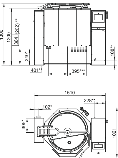
КПЭМ-250-ОМП, КПЭМ-350-ОМП
