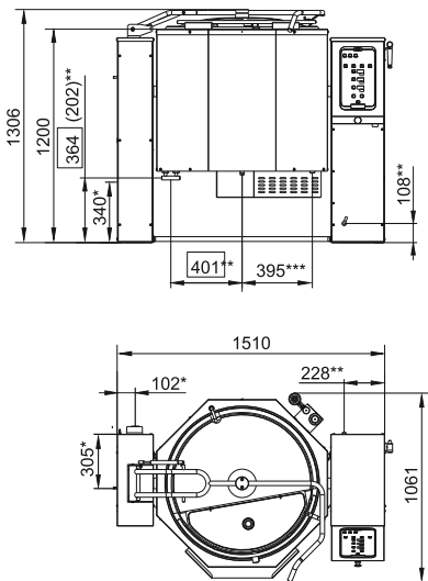
КПЭМ-250-0М2, КПЭМ-350-0М2
