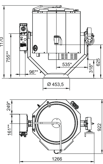
КПЭМ-100-ОМР
