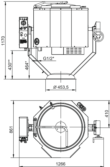
КПЭМ-100-ОМР
