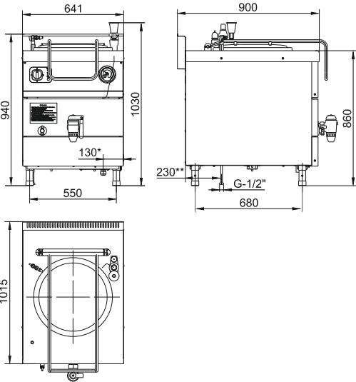
КПЭМ-60/9Т
