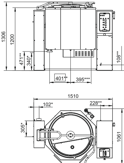
КПЭМ-200-0М2
