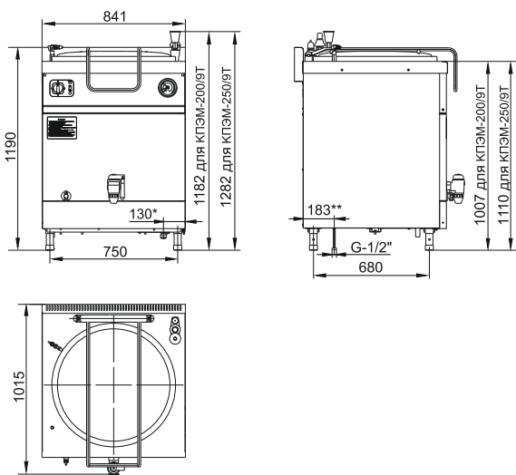
КПЭМ-200/9Т, КПЭМ-250/9Т
