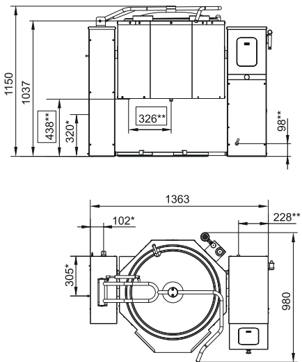
КПЭМ-100-0
