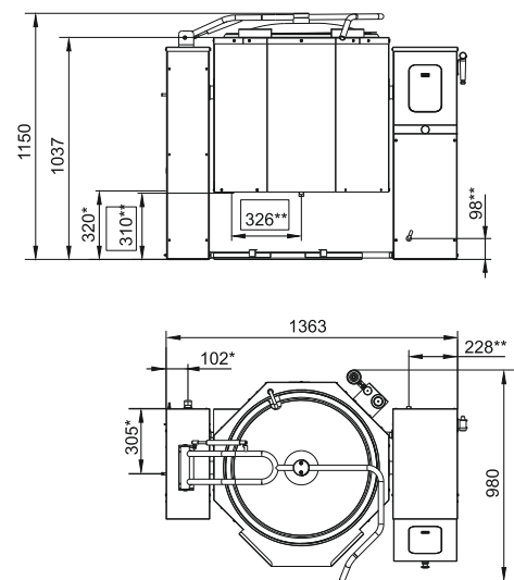
КПЭМ-160-0
