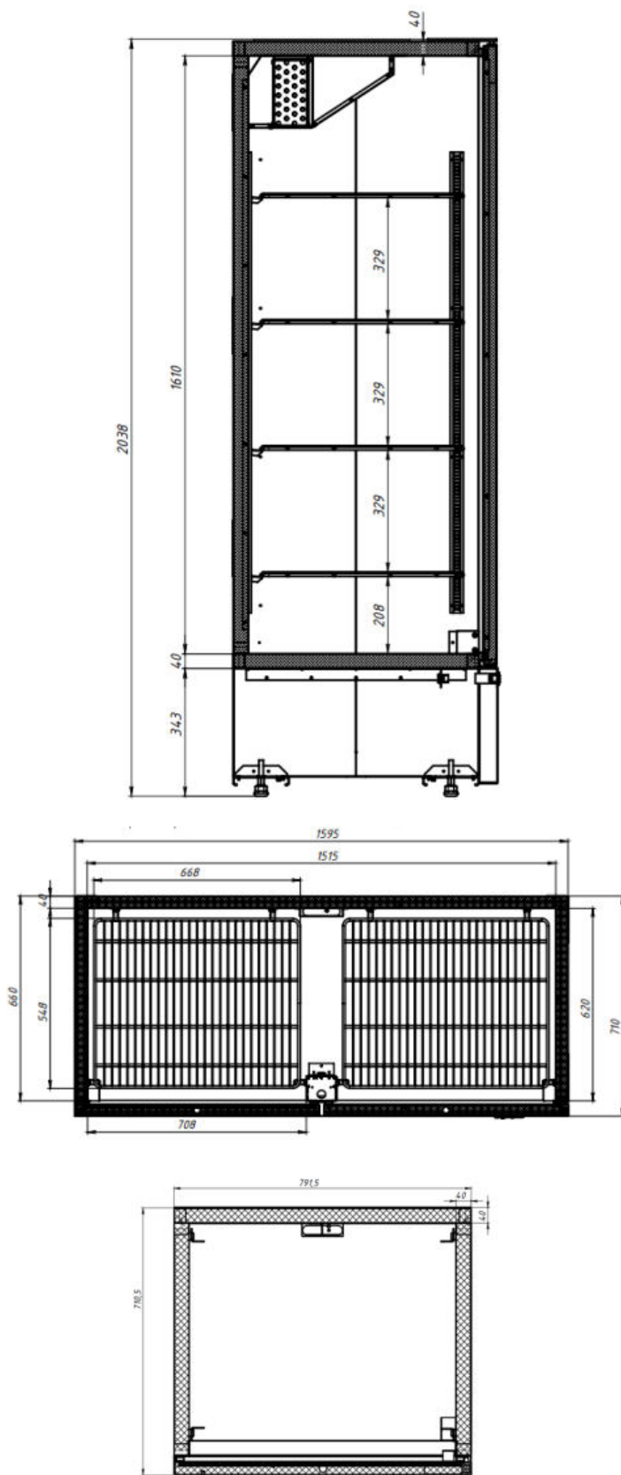
рисунок 2 – Сечение шкафа холодильного «Shkaff CT 1400 и 700»
