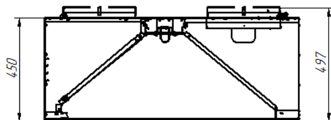
а) ЗПВ-900-1,5П
