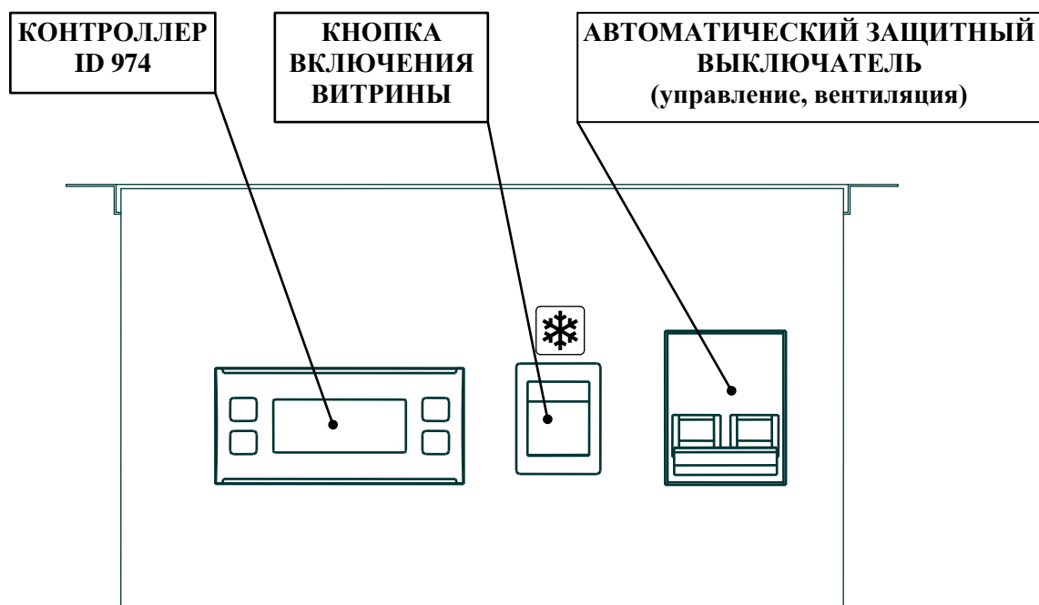
Рис. 2. Блок управления витрины «ВИЛИЯ» Б ВС
