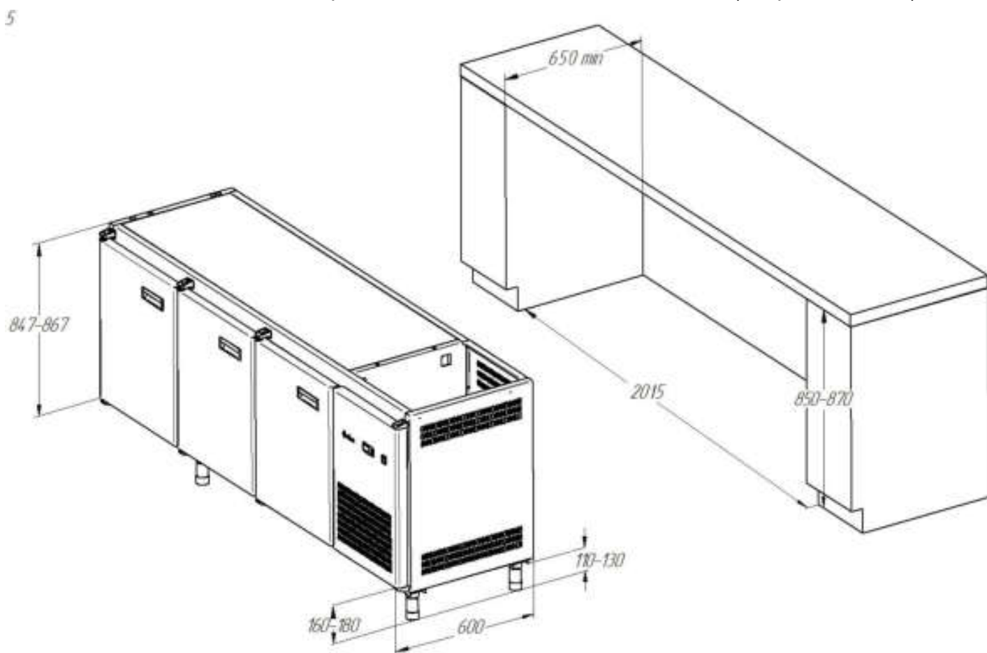
Рис.26. Схема встраивания CXH-60-02 без столешницы (дверь, дверь, дверь).
