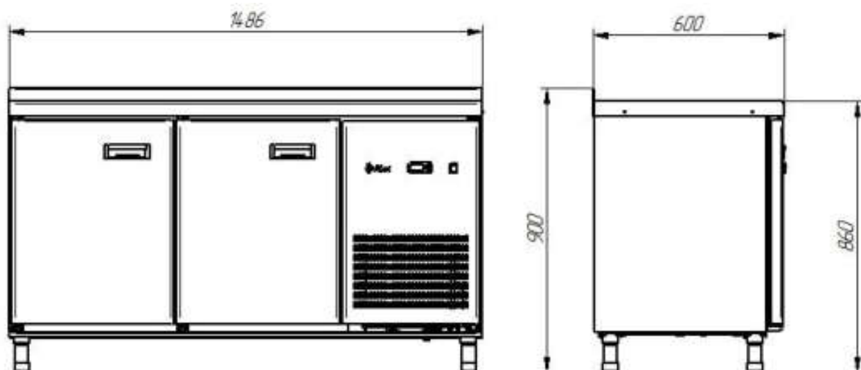
Рис.14. Габаритные размеры CXH-60-01 столешница с бортом (дверь, дверь)*
