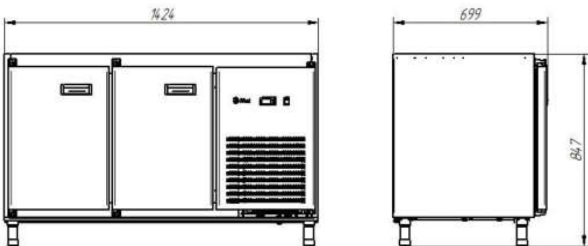
Рис.6. Габаритные размеры CXH-70-01 столешница без борта (дверь, дверь)*
