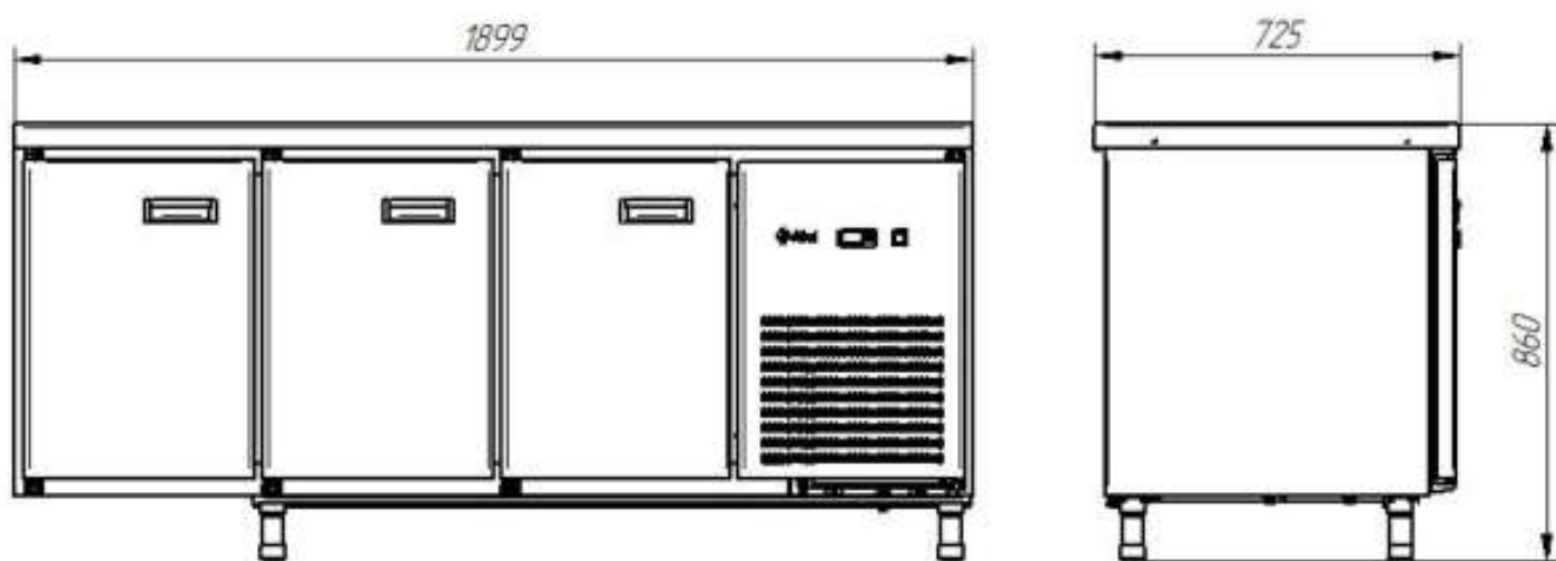
Рис.9. Габаритные размеры CXH-70-02 столешница без борта (дверь, дверь, дверь)*
