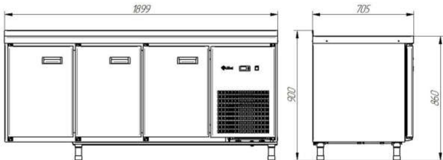
Рис.8. Габаритные размеры CXH-70-02 столешница с бортом (дверь, дверь, дверь)*
