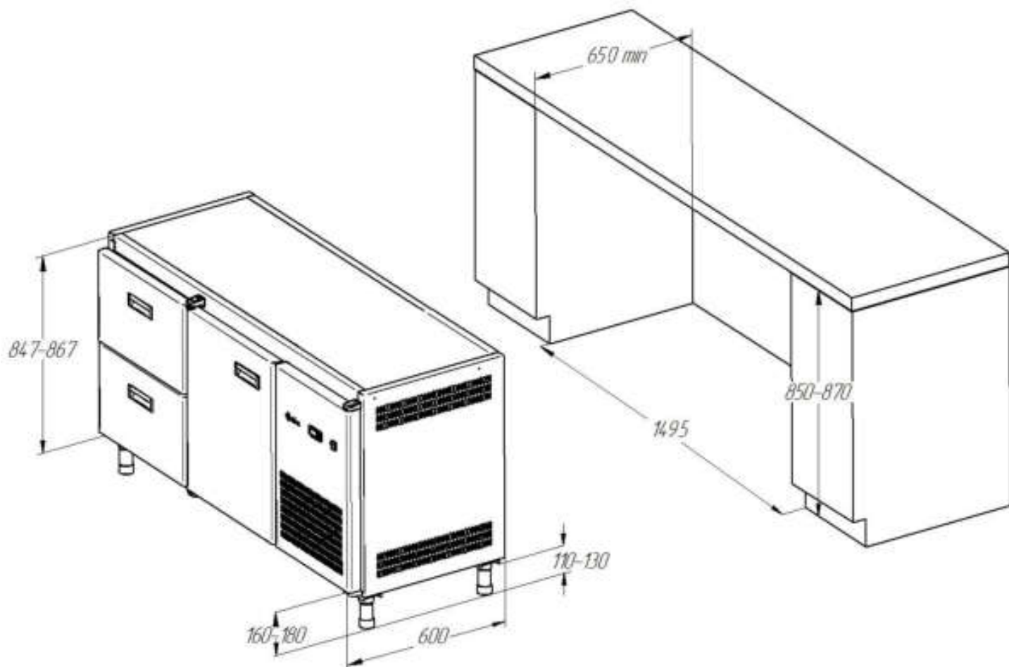
Рис.25. Схема встраивания CXH-60-01 без столешницы (дверь, ящики 1/2).
