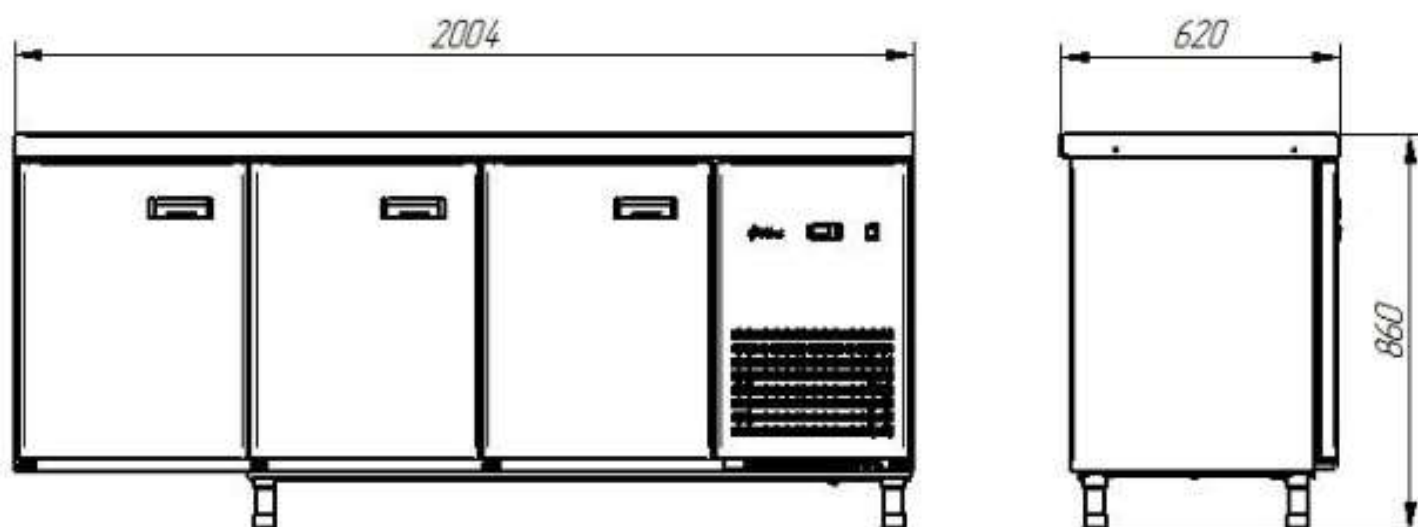
Рис.17. Габаритные размеры CXH-60-02 столешница с бортом (дверь, дверь, дверь)*
