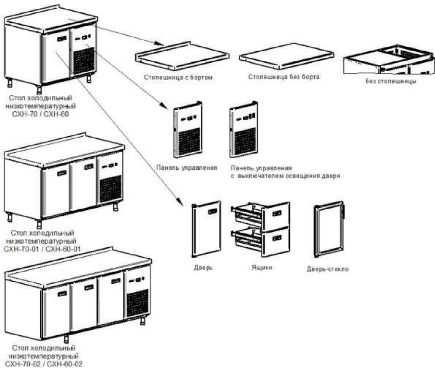
Рис.1. Варианты исполнений CXH-70; CXH-60; CXH-70-01; CXH-60-01; CXH-70-02; CXH-60-02.
