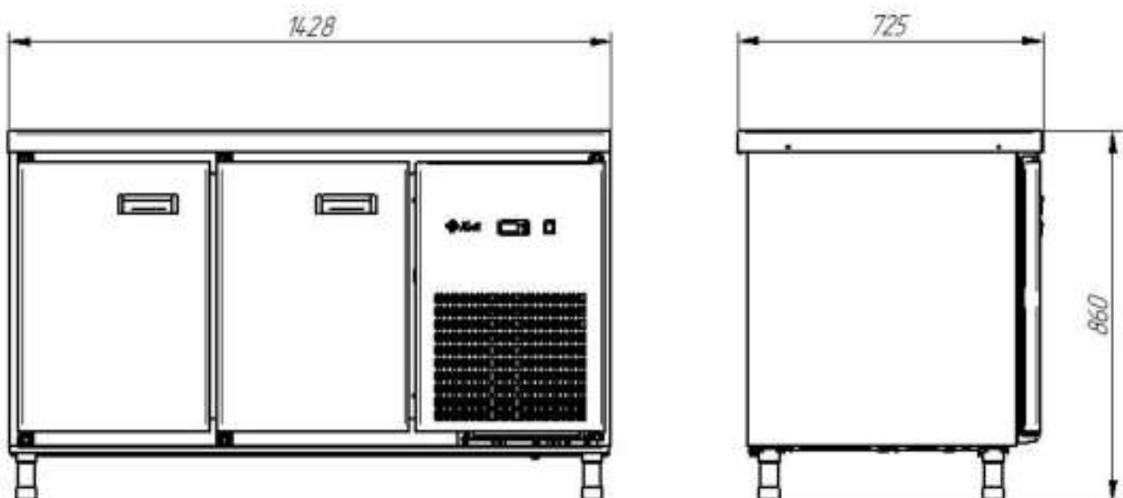
Рис.6. Габаритные размеры CXH-70-01 столешница без борта (дверь, дверь)*
