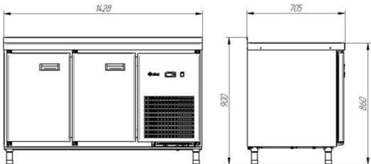
Рис.5. Габаритные размеры CXH-70-01 столешница с бортом (дверь, дверь)*
