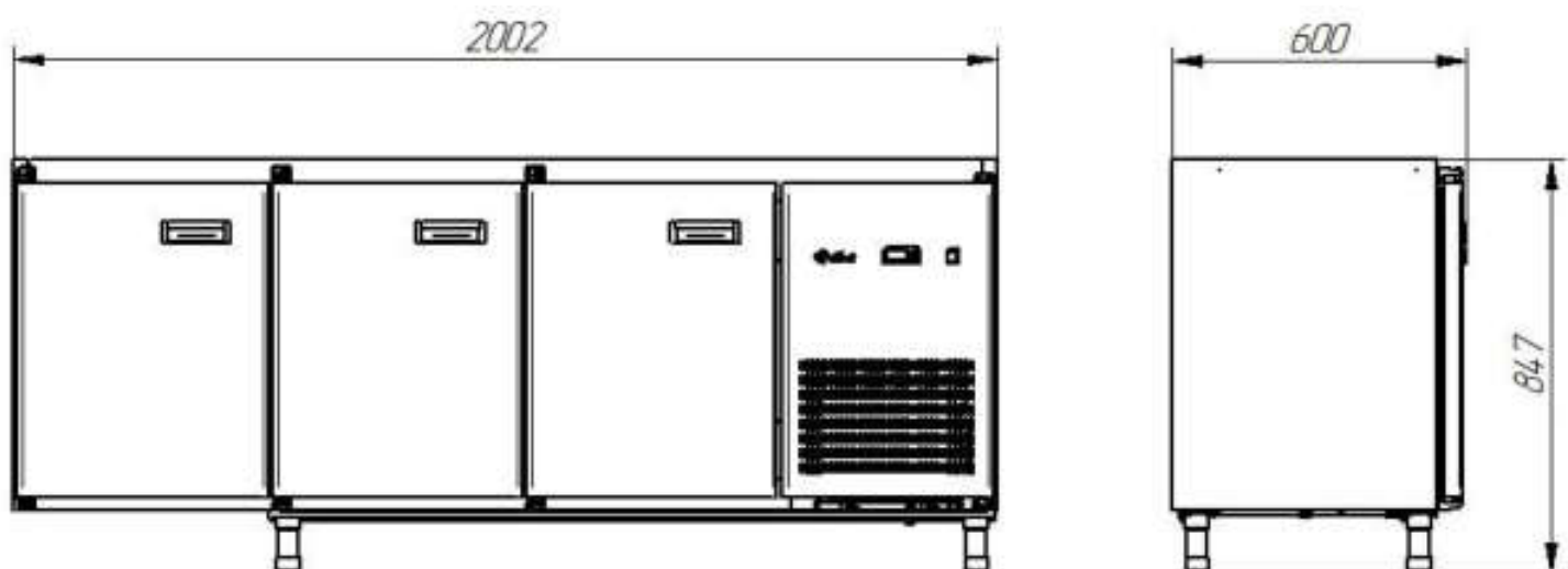
Рис.18. Габаритные размеры CXH-60-02 столешница без борта (дверь, дверь, дверь)*
