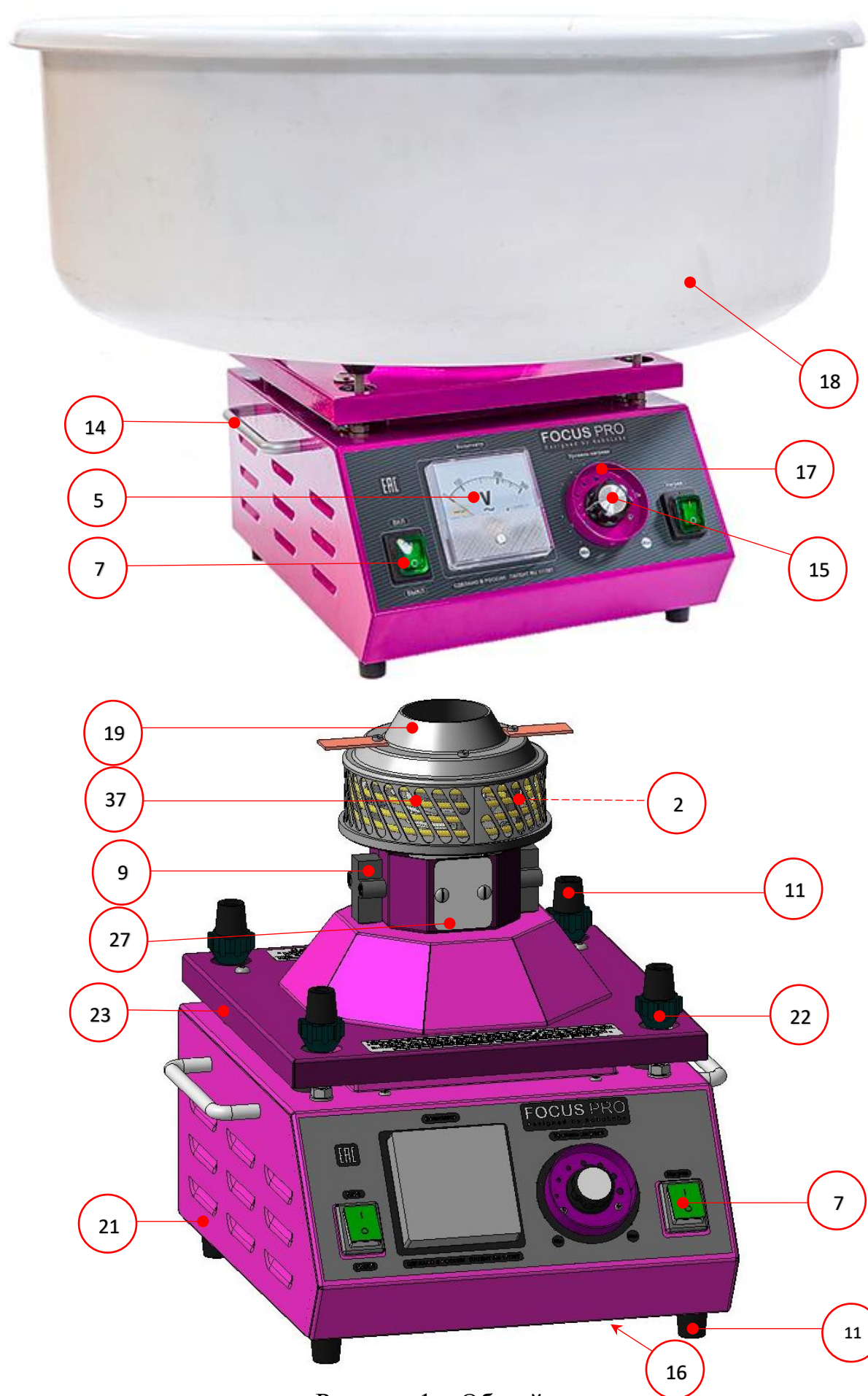
Рисунок 1 – Общий вид
