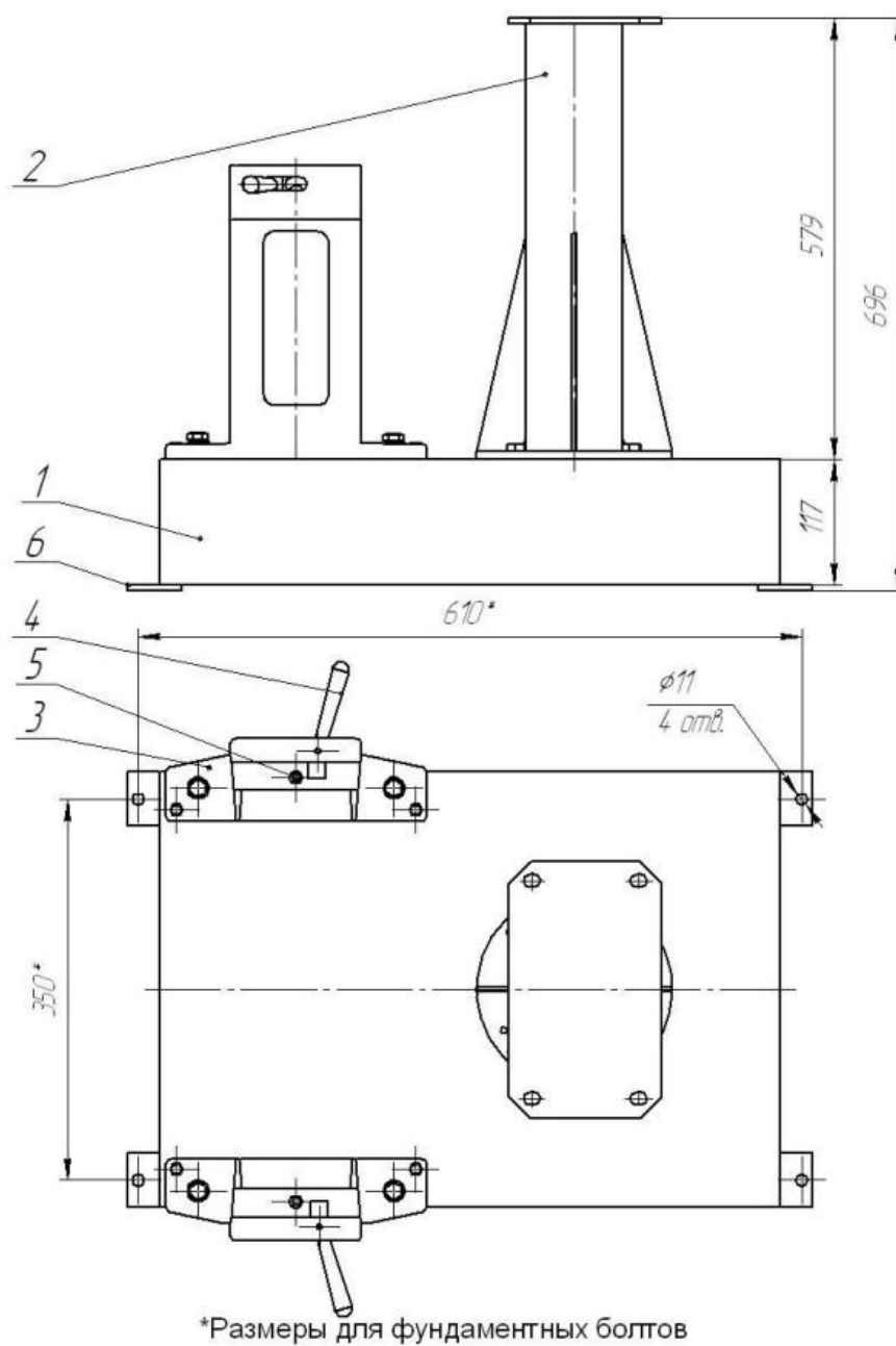
Рисунок – 8 Подставка
